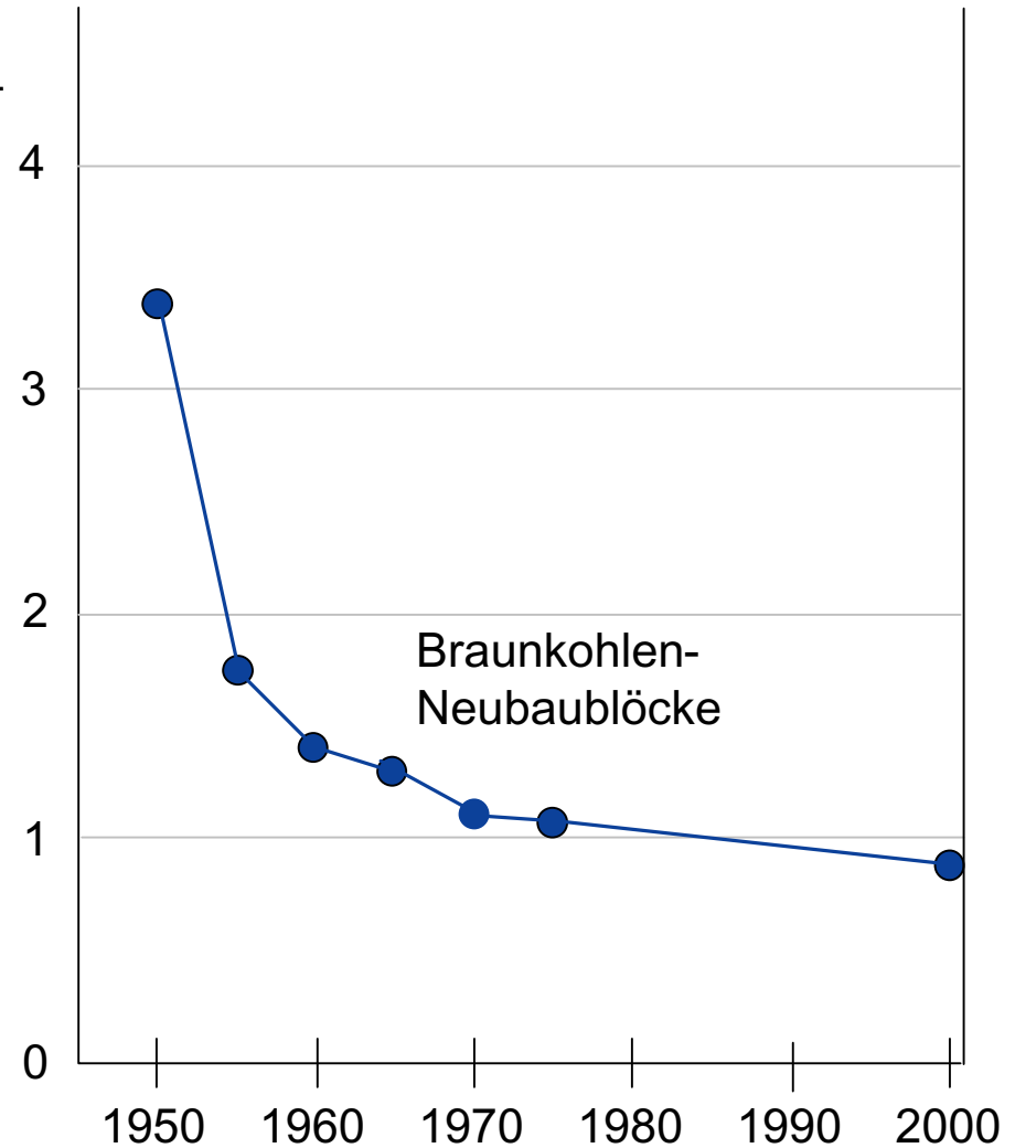
Spezifische CO 2 -Emissionen in kg/kWh
